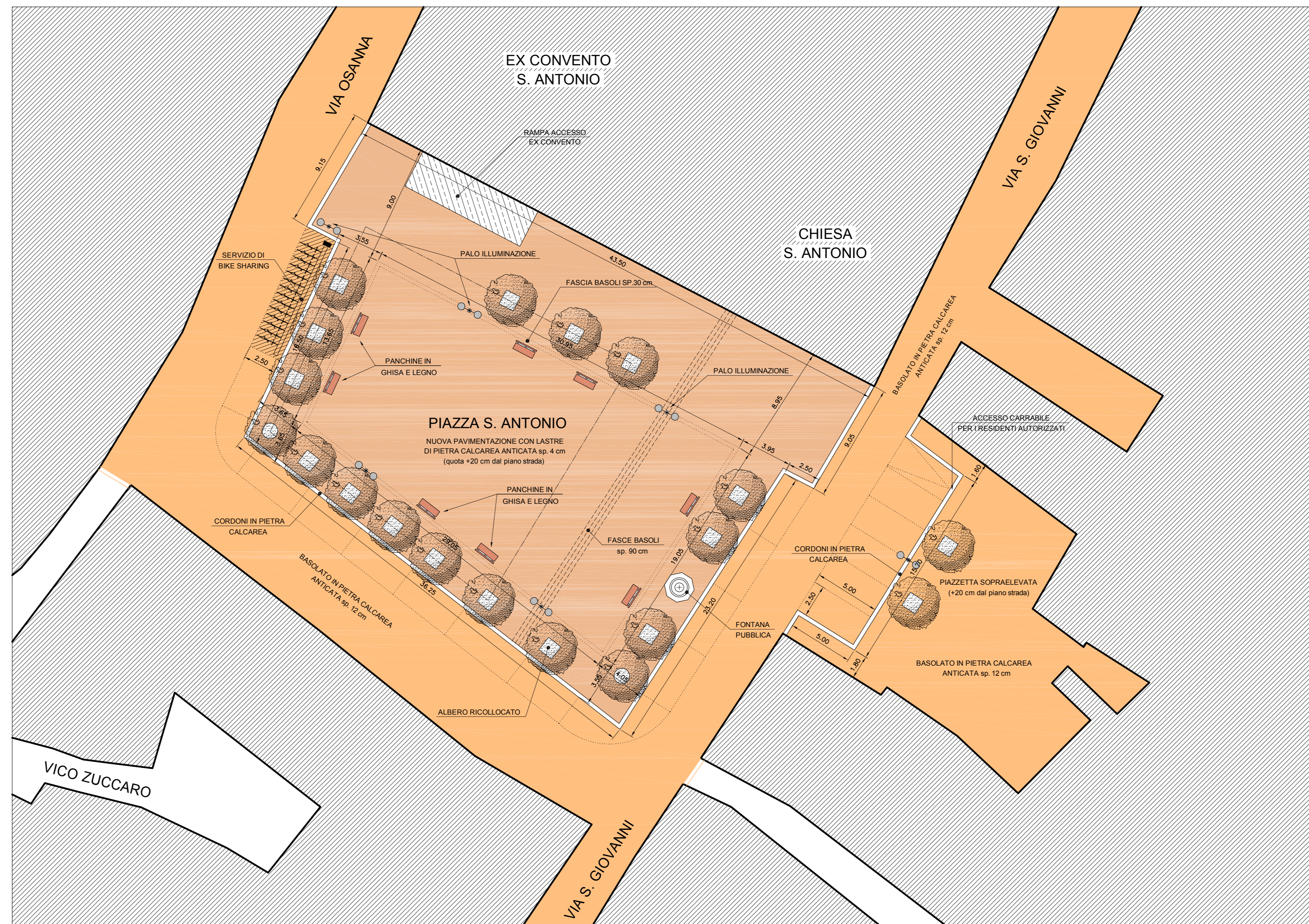
PLANIMETRIA DI PROGETTO PIAZZA S. ANTONIO
